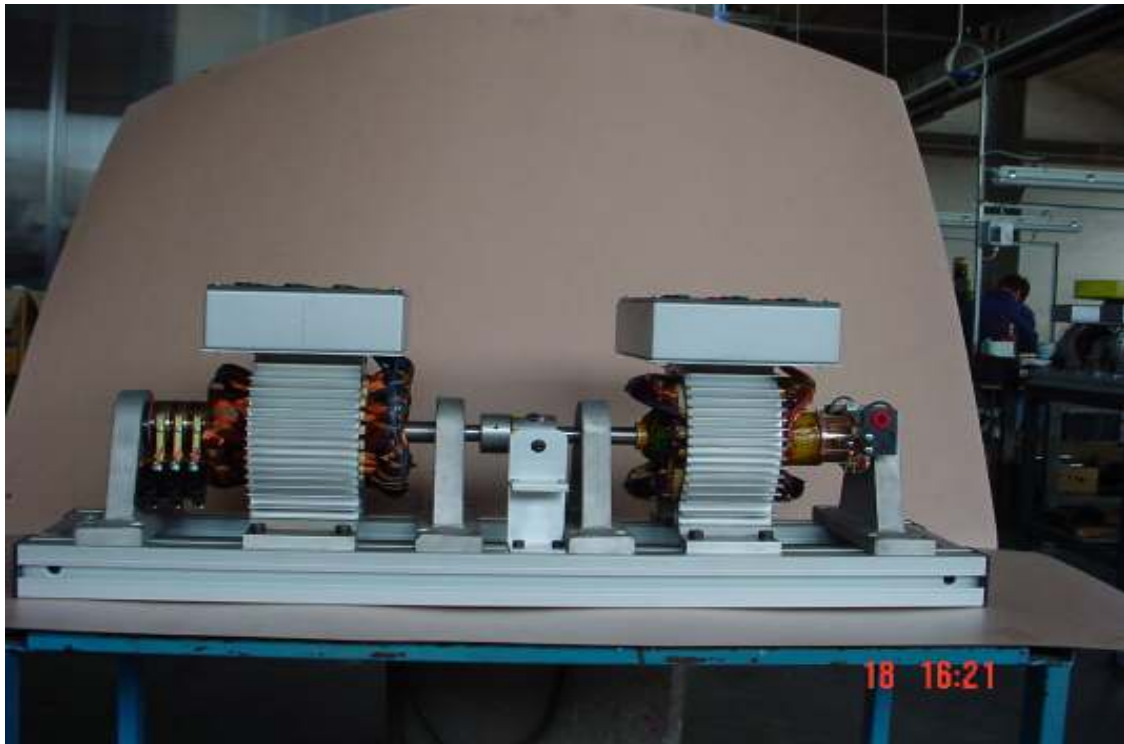
Motori in Corrente Continua ed in Corrente Alternata in versione aperta per uso didattico con montaggio su basamento di accoppiamento.
